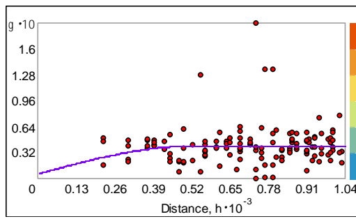
pH
