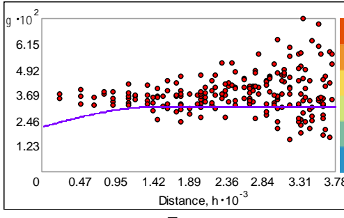
Zn
