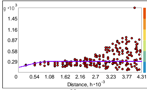
Mn
