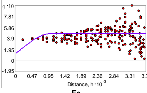
Fe
